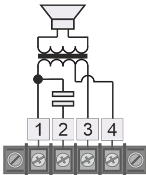
Рисунок 2. Схема громкоговорителя
