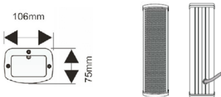
Рисунок 1. Внешний вид громкоговорителя
