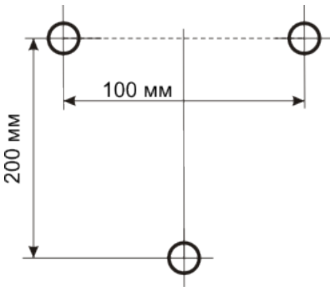
Рисунок 1. Крепление настенного громкоговорителя
