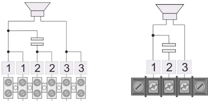
Рисунок 2. маркировка клемм подключения
